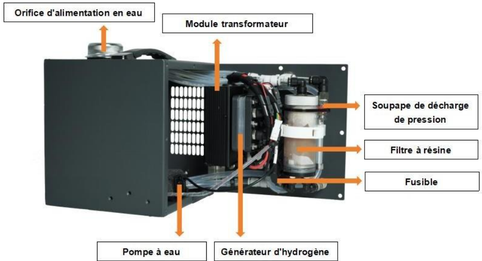
Structure interne du système
